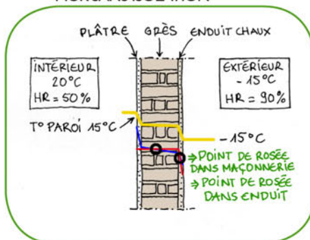
MUR SANS ISOLATION
