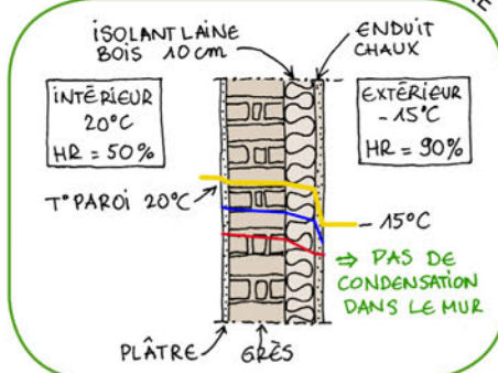
MUR AVEC ISOLATION EXTERIEURE
