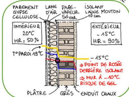
MUR AVEC ISOLATION INTERIEURE
